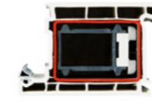
Renfort acier galvanisé 2 mm pour 70 mm 3 mm pour 82 mm
