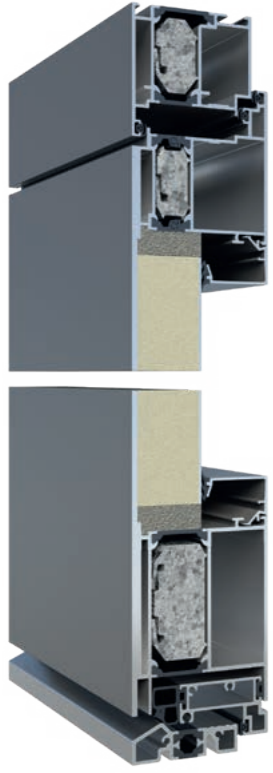
Abb. flügelüberdeckende Füllung außen (Mehrpreis)
